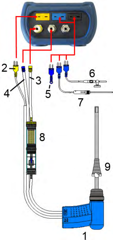
Bild 1: Anschlussschema (Sensorseite)
