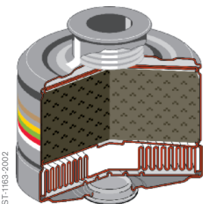
Dräger X-plore® Rd40 Filter: Schnittzeichnung
